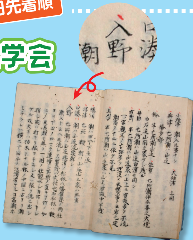
宝永地震の被害記録(「谷陵記」)
